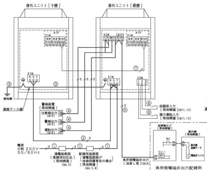
【電源が庫外ユニット～庫外ユニットを渡る場合】
