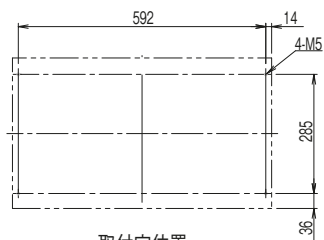
取付穴位置
